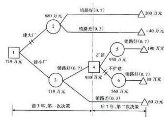
图 9-4 例 9.7 的决策树
